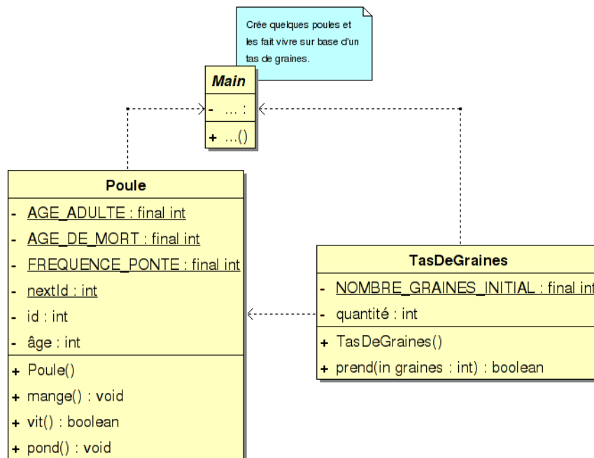
FIG. 1 – Diagramme UML
